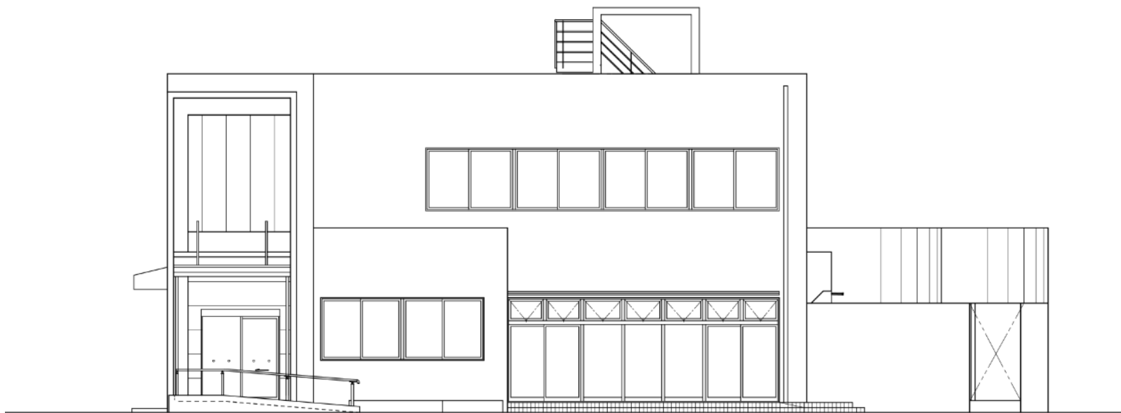
西側立面図
