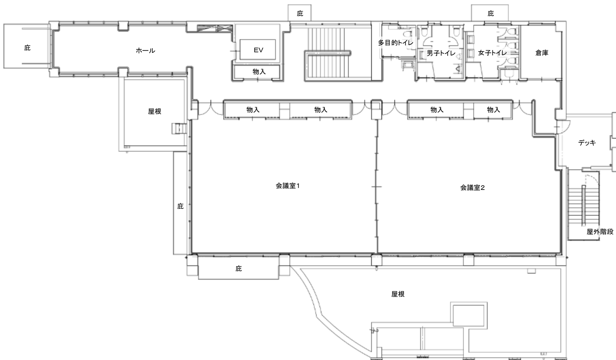
2 階 平 面 図
