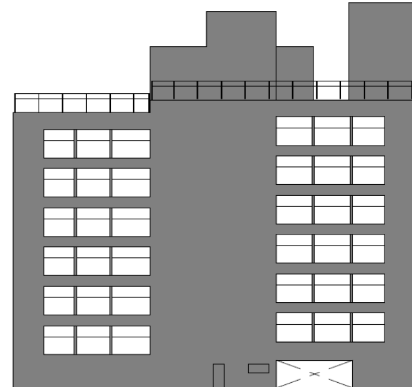
西側立面図
