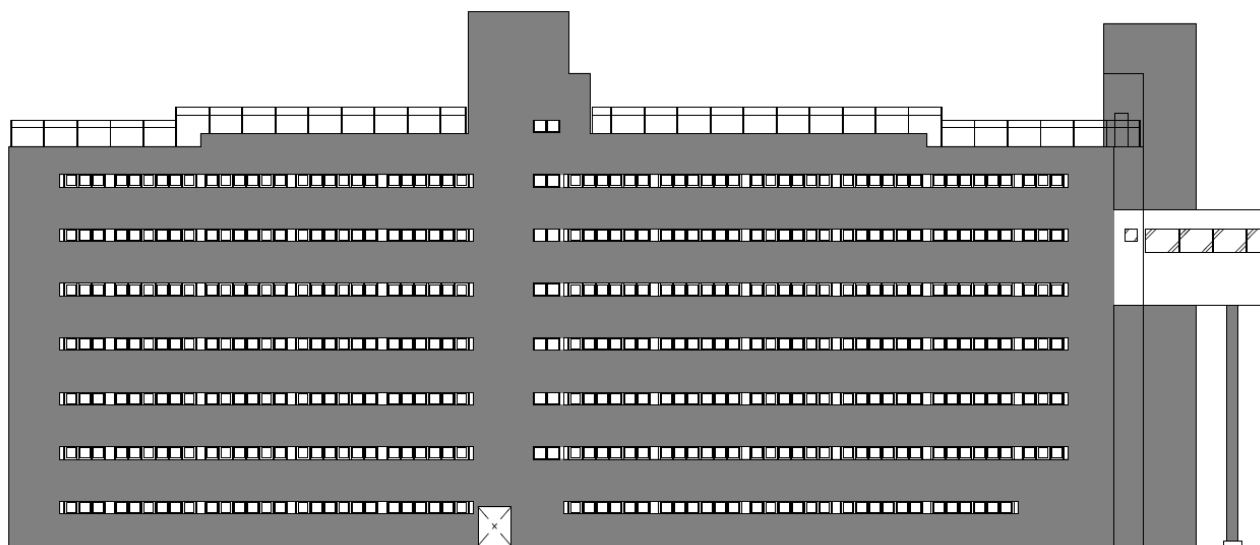
南側立面図
