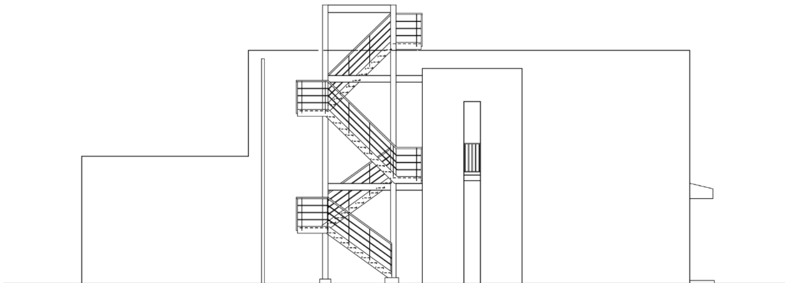
東側立面図
