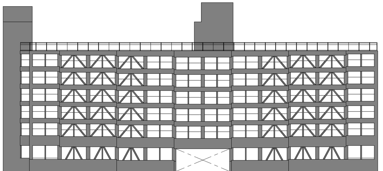
北側立面図
