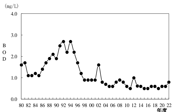
図1-3 BODの経年変化(十王川)
