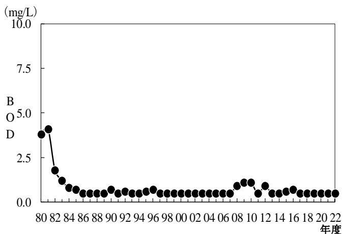
図1-7 BODの経年変化(鮎川)
