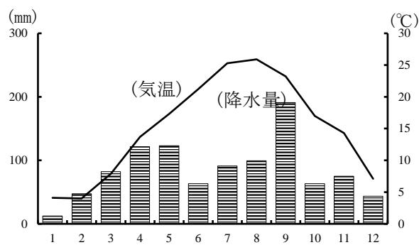
図1-2 気温と降水量の月変化 (2022年日立市役所観測所)
