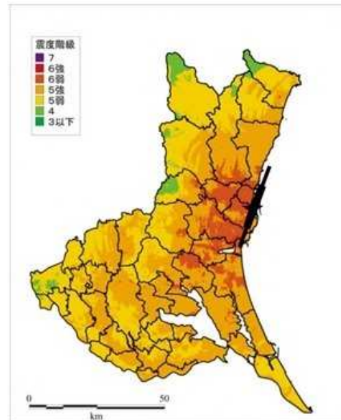
図2 太平洋プレート内の地震（北部）の 地表震度分布 出典：茨城県地震被害想定調査 詳細報告書
