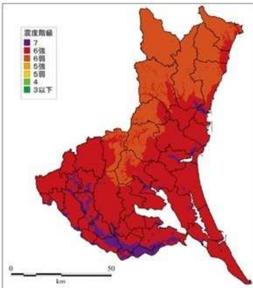
図3 地殻内に一律にMw6.8の震源を 想定した場合の震度分布 出典：内閣府 地震防災マップ作成技術資料を基に作成
