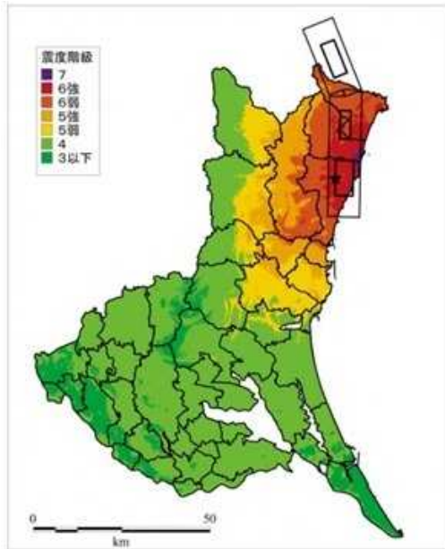
図1 F1断層などの連動の地震の 地表震度分布 出典：茨城県地震被害想定調査 詳細報告書
